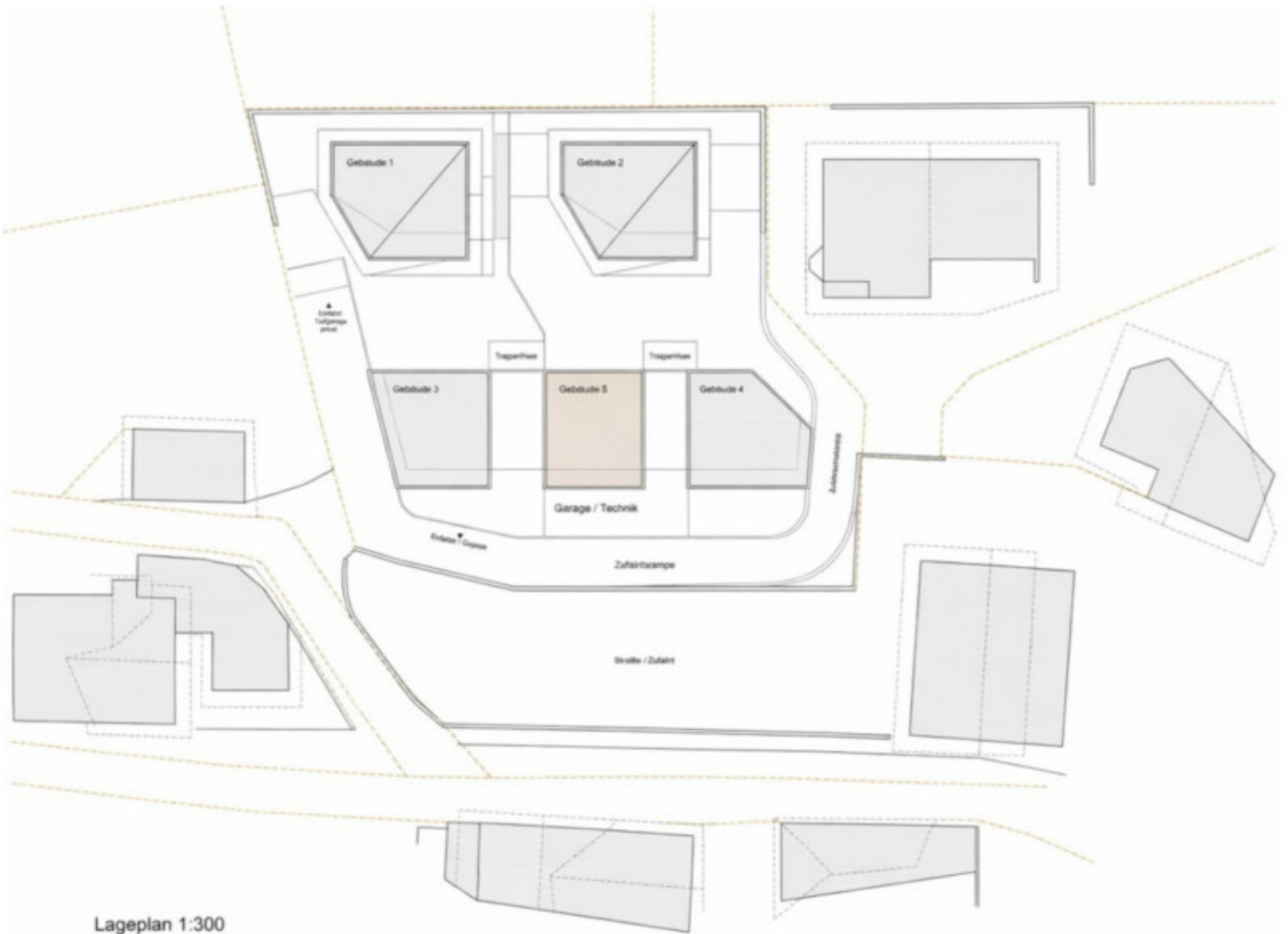
Lageplan 1:300
