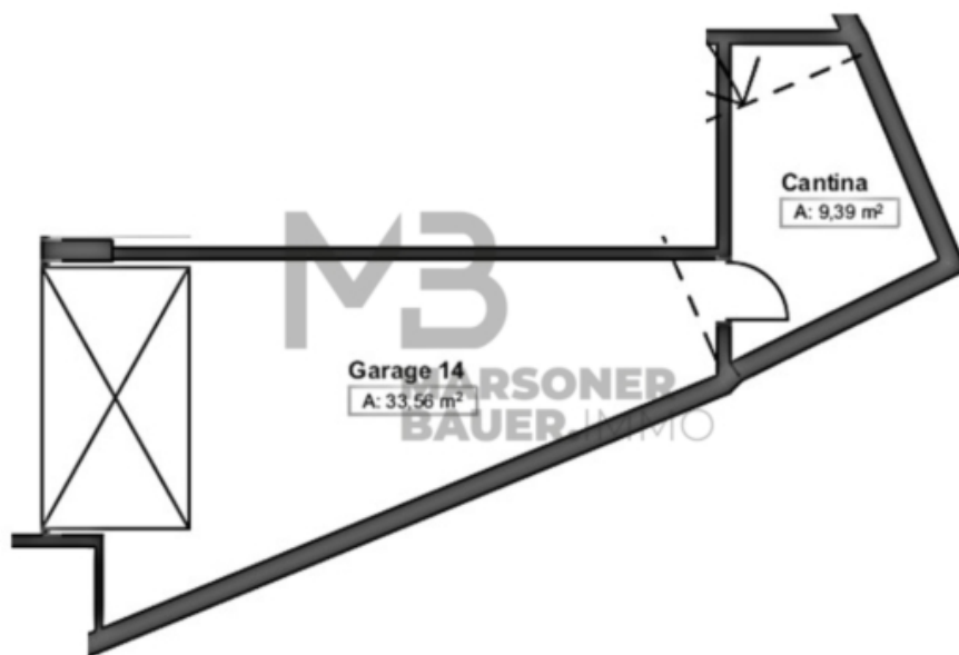
PIANO INTERRATO / UNTERGESCHOSS
