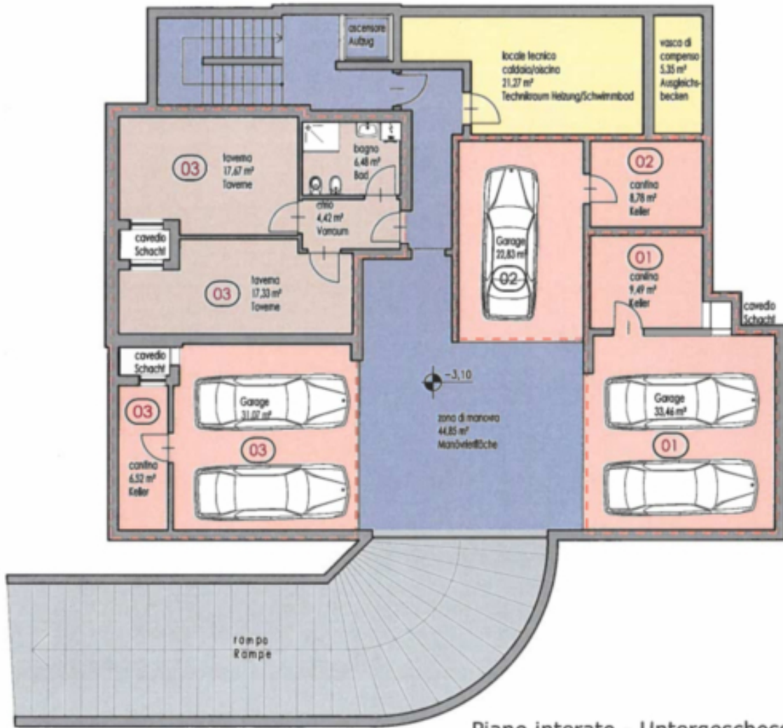
Piano interato - Untergeschoss
