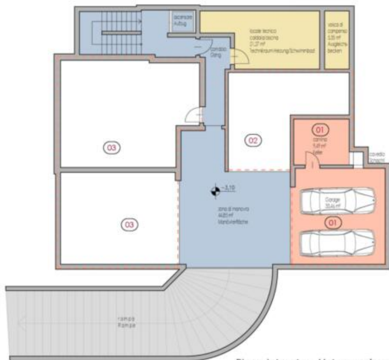
Piano interato - Untergeschoss
