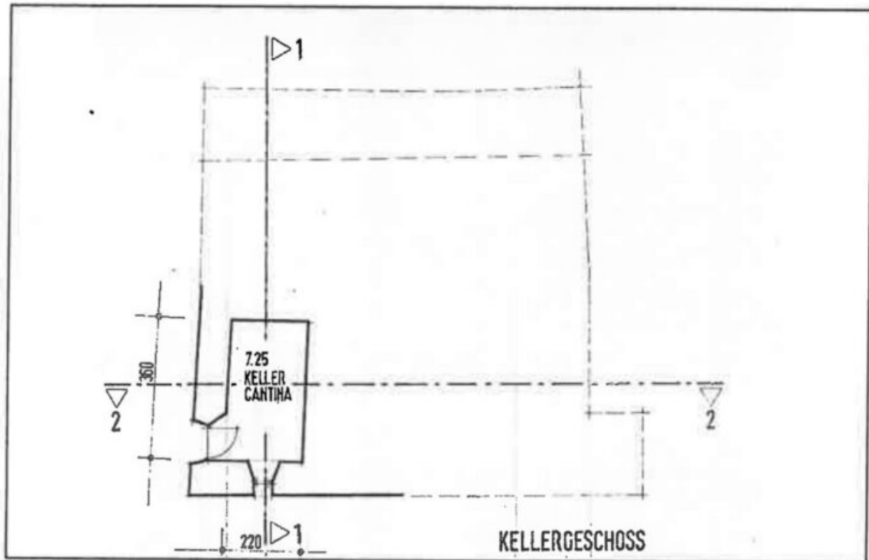
GRUNDRISS KELLERGECHOSS
