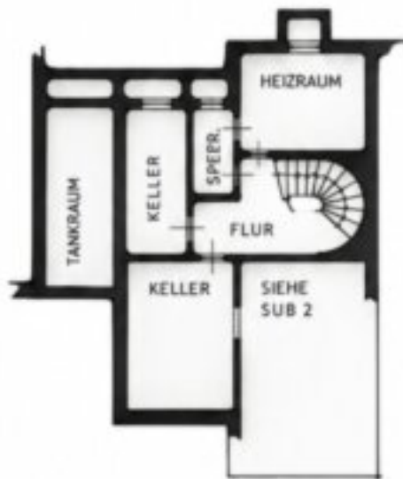
KELLERGESCHOSS SCANTINATO H2.50
