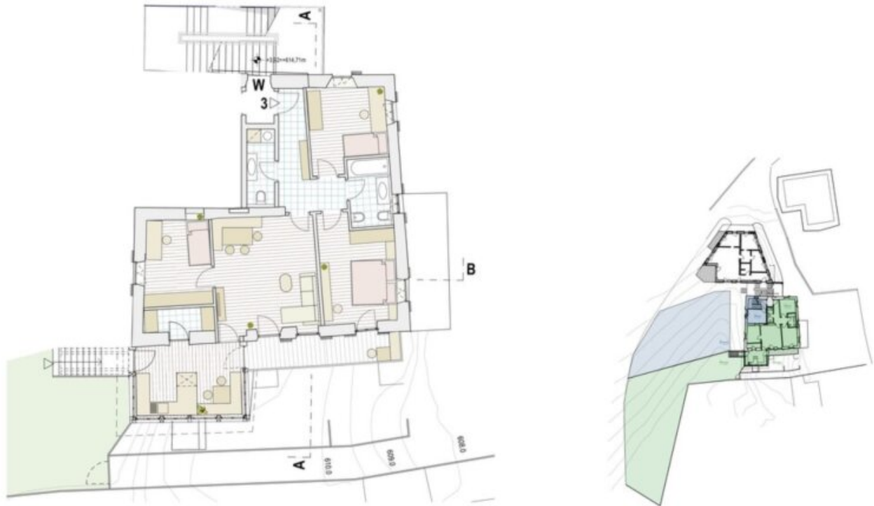
Wohnung 3 M1-500, 1:100
