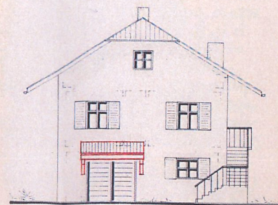
SÜDANSICHT
