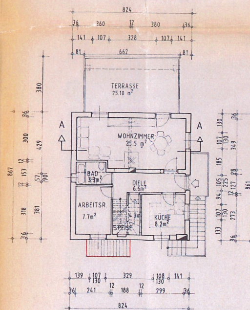
GRUNDRIS OBERGESCHOSS
