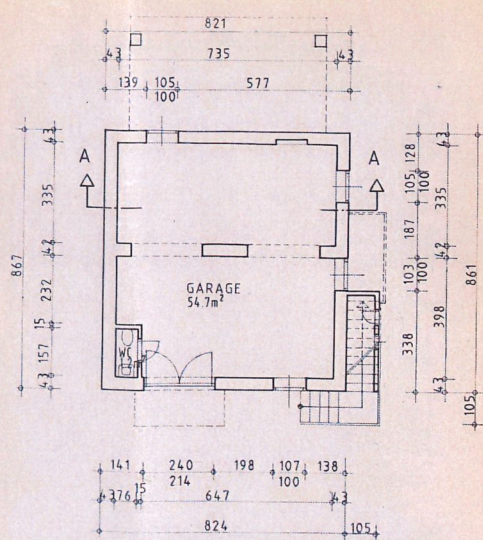
GRUNDRIS ERDGESCHOSS
