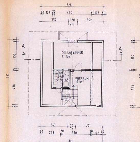
GRUNDRIS DACHGESCHOSS
