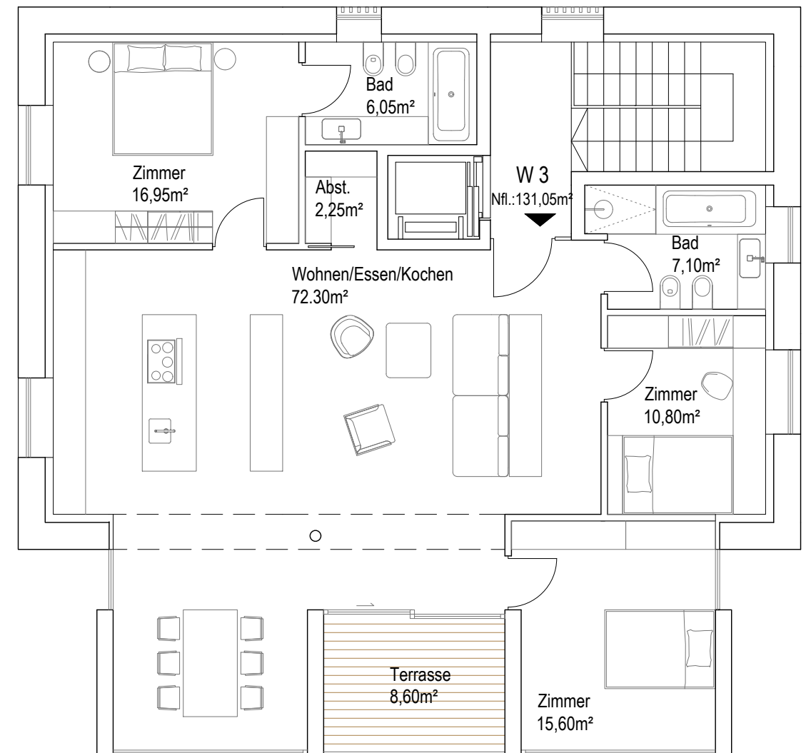
2. OBERGESCHOSS 1:100
