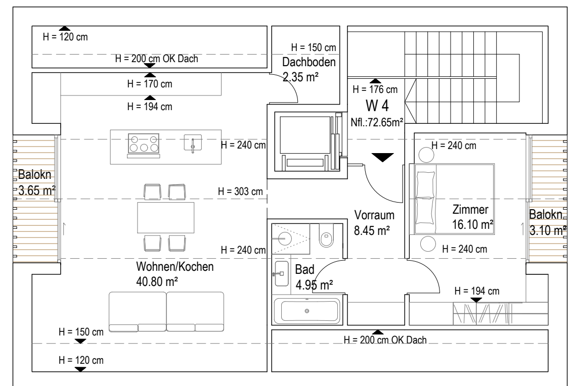
DACHGESCHOSS 1:100
