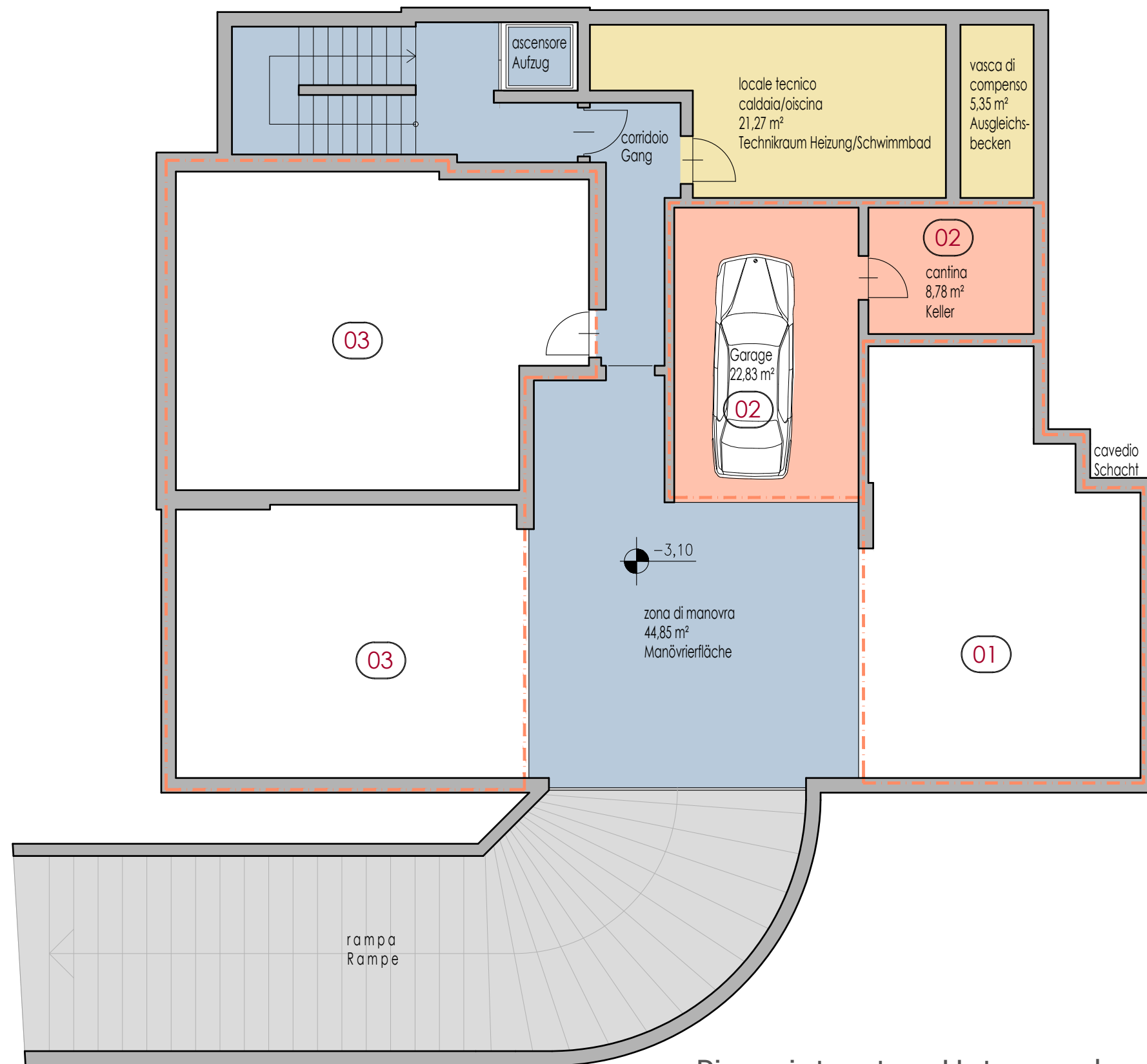
Piano interato - Untergeschoss
